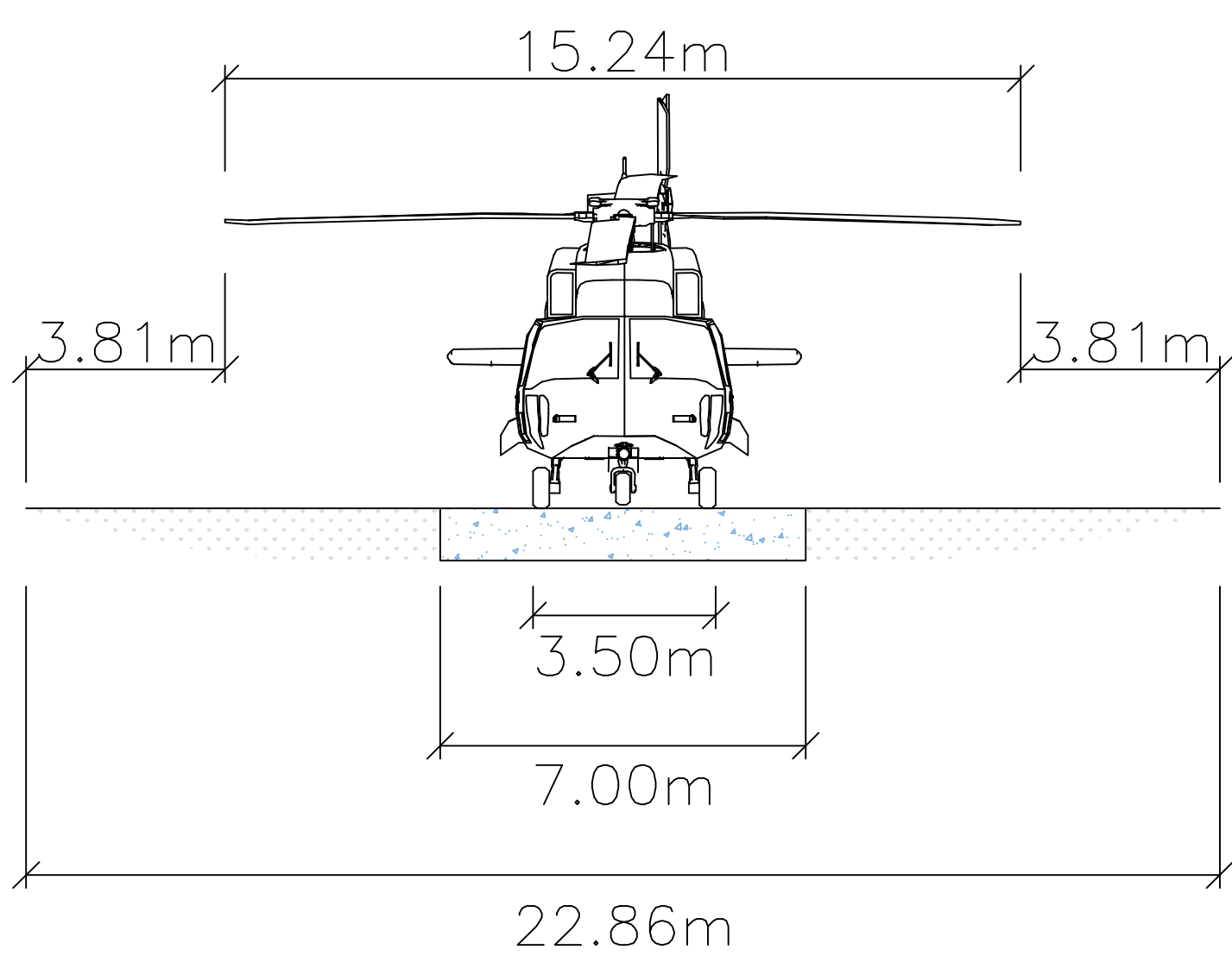
PISTA E ROTA DE TÁXI TERRESTRE – VISTA ESCALA 1:125
