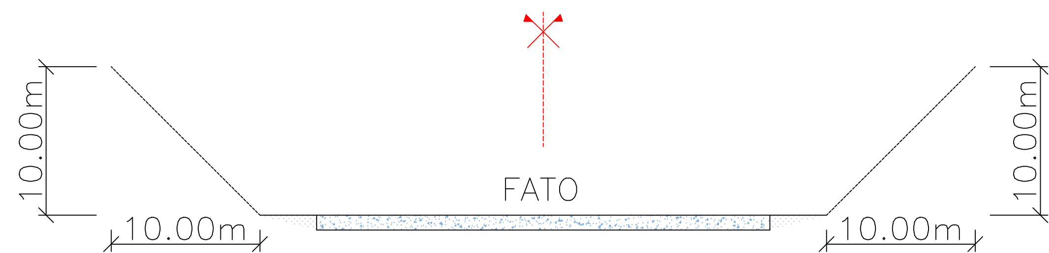
RAMPA LATERAL PROTEGIDA – CORTE AA ESCALA 1:250
