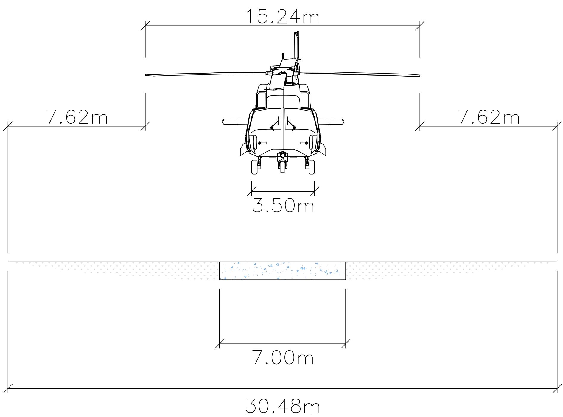
PISTA E ROTA DE TÁXI AÉREO – VISTA ESCALA 1:125
