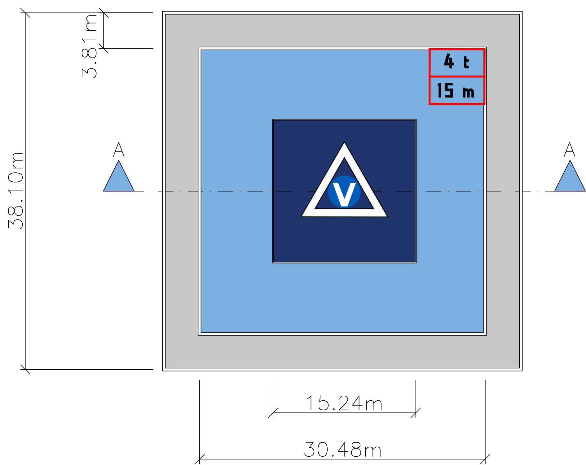
FATO E ÁREA DE SEGURANÇA ASSOCIADA – PLANTA ESCALA 1:250
